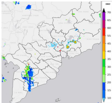
Hình 1: Ảnh ra đa thời tiết tại khu vực Nam Bộ
